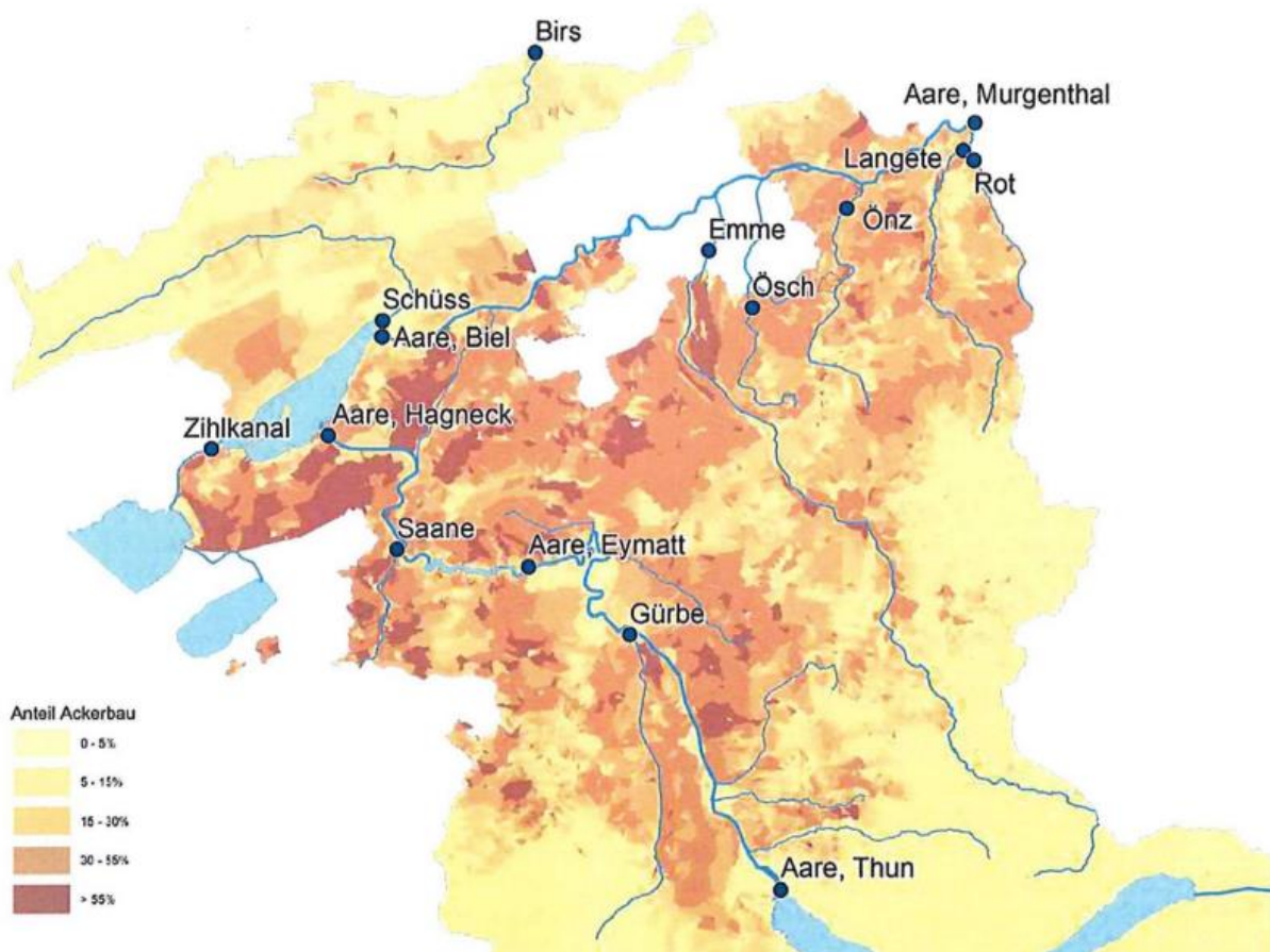
Fig. 1 Darstellung der untersuchten Oberflächengewässer und Probenahmestandorte im Kanton Bern, bei denen 2020 anhand monatlicher Stichproben die beiden Chlorothalonil-Metaboliten R417888 und R471811 gemessen wurden.
