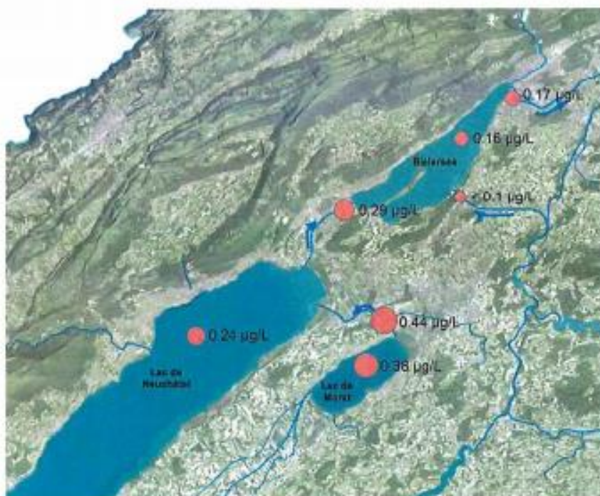
Fig. 6 Gemessene Konzentrationssummen (R417888 und R471811) im Seeverbund Bieler-, Neuenburger- und Murtensee der Stichproben vom März 2020. Die blauen Pfeile geben die Fliessrichtungen der Verbindungsgewässer an.
