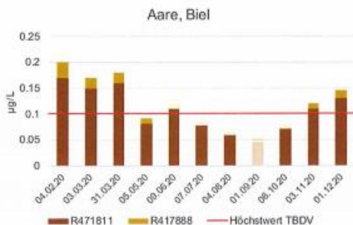
Fig. 5 Gemessene Konzentrationen der Chlorothalonil-Metaboliten R417888 (orange) und R471811 (dunkelrot) in der Aare beim Auslauf des Bielersees. Bei den transparent dargestellten Konzentrationen lagen die Werte knapp unter den festgesetzten Bestimmungsgrenzen gemäss Tab. 1, konnten jedoch trotzdem mit ausreichender Verlässlichkeit quantifiziert werden.
