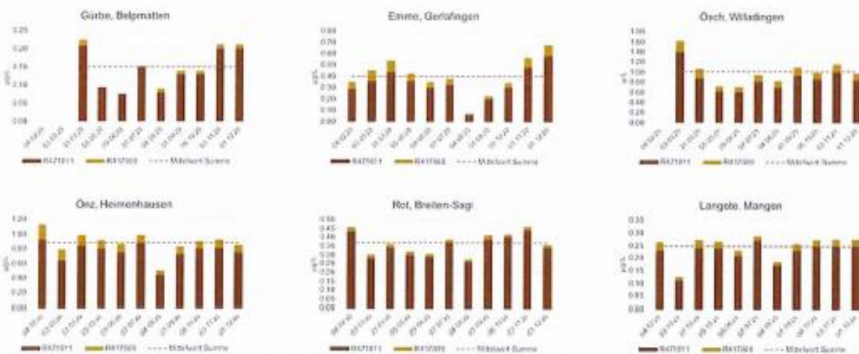
Fig. 4 Gemessene Konzentrationen der Chlorothalonil-Metaboliten R417888 (orange) und R471811 (dunkelrot) in den Aare-Zuflüssen. Dargestellt ist zudem der jeweilige Mittelwert der Konzentrationssumme beider Metaboliten über die gesamte Messperiode (gestrichelte Linie). In der Gürbe wurde die Probenahme erst Ende März, in der Ösch Anfang März gestartet. Unterschiedliche Skalierung der Konzentrationen auf den y-Achsen.
