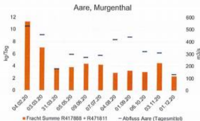
Fig. 3 Tagesfracht der Summe der Chlorothalonil-Metaboliten R417888 und R471811 in der Aare bei Murgenthal. Als blauer Balken dargestellt ist der Abfluss der Aare (Tagesmittel) zum Zeitpunkt der Probenahme.
