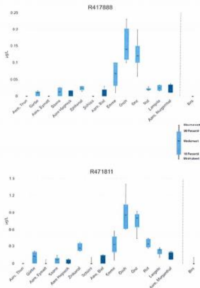
Fig. 2 Gemessene Konzentrationen der Chlorothalonil-Metaboliten R417888 (oben) und R471811 (unten). Die Messstellen wurden entlang der Fliessrichtung der Aare angeordnet. Die fünf Aare-Messstellen sind in Dunkelblau dargestellt, die übrigen Gewässer in Hellblau. Die Konzentrationen auf den y-Achsen sind unterschiedlich skaliert.
